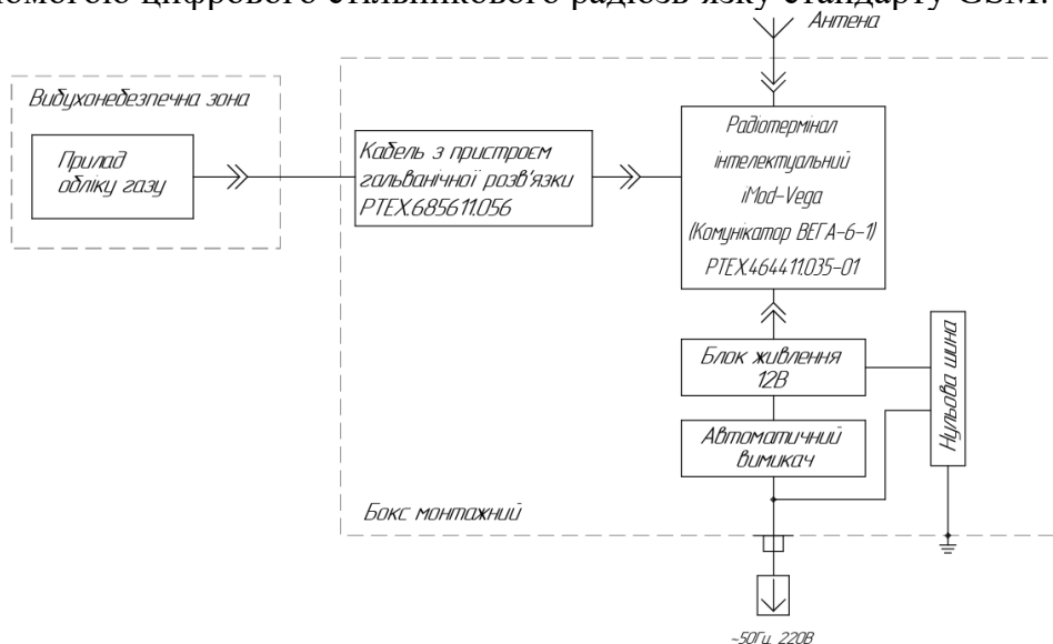
Рисунок 1 – Схема підключення модулю
