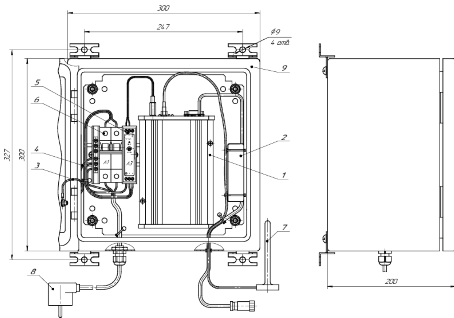
Рисунок 2 – Зовнішній вигляд, габаритні та приєднувальні розміри модуля
